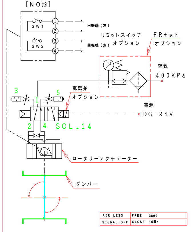
フローシート図 [TA2-0402D-□□-□□□]
